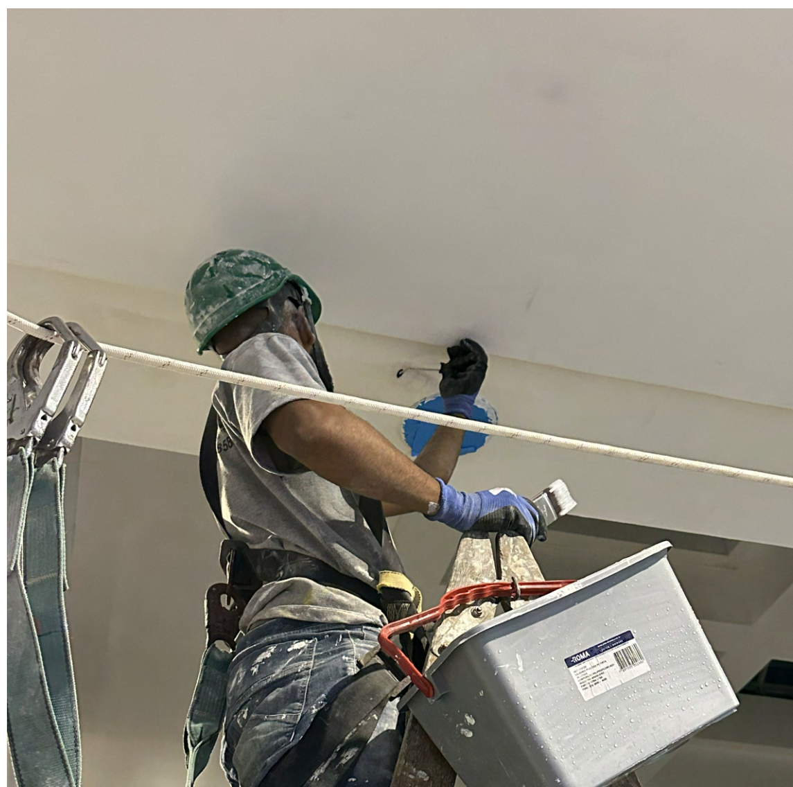
Reparo no forro em drywall, construção de parede e instalação de divisórias Eucatex
