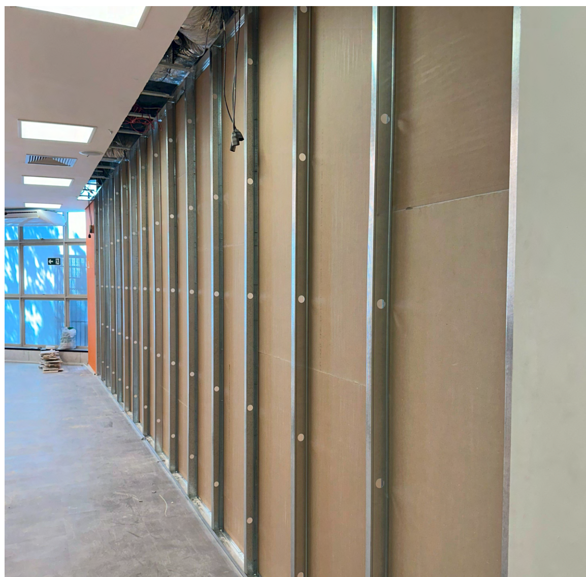
Instalação de parede em drywall
